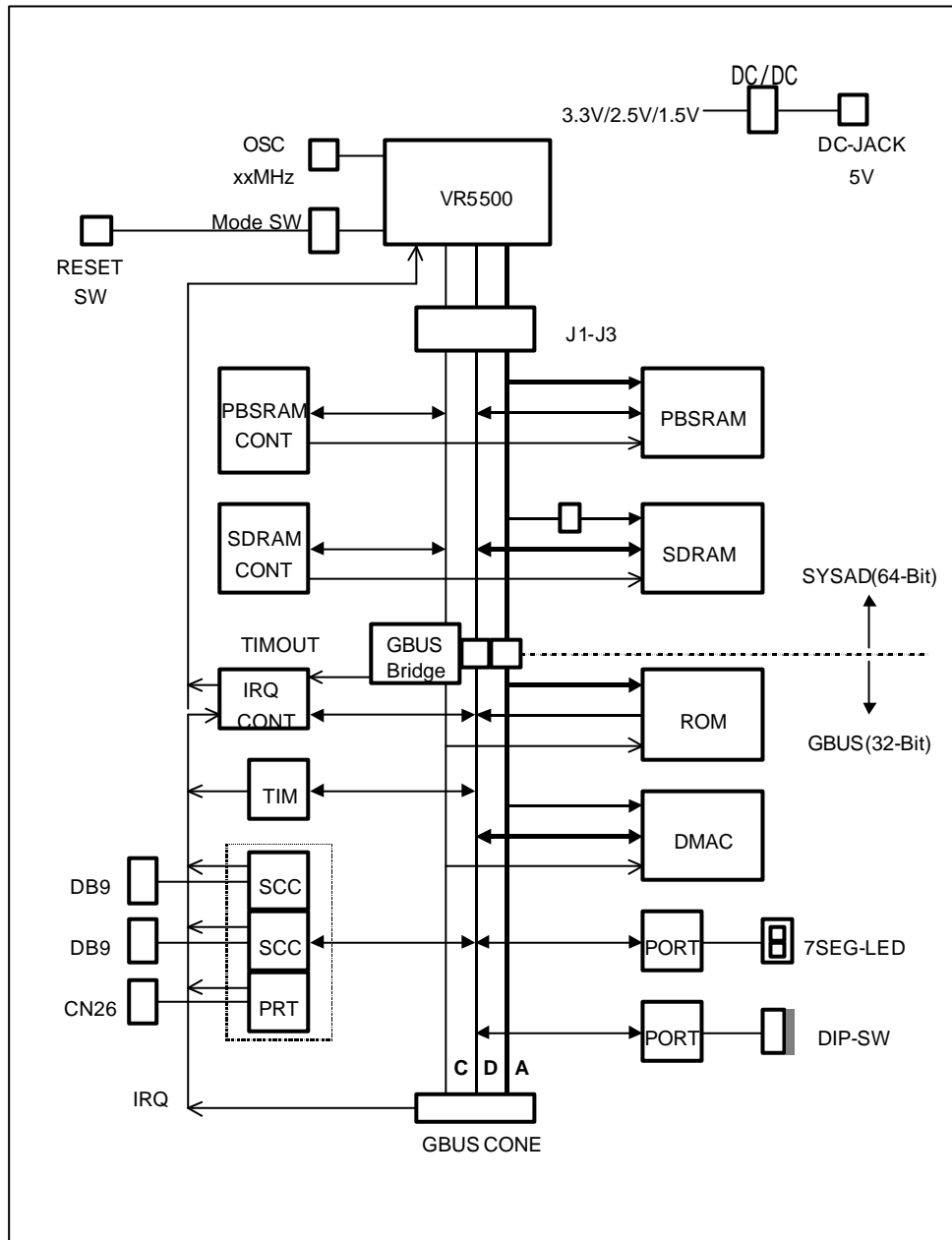
ブロック図
