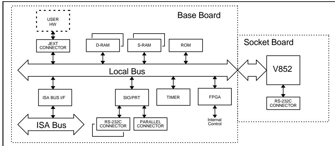
RTE-V852-PC Block Diagram
