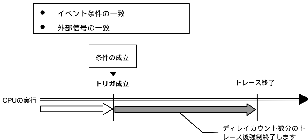
図 10 トリガ条件
